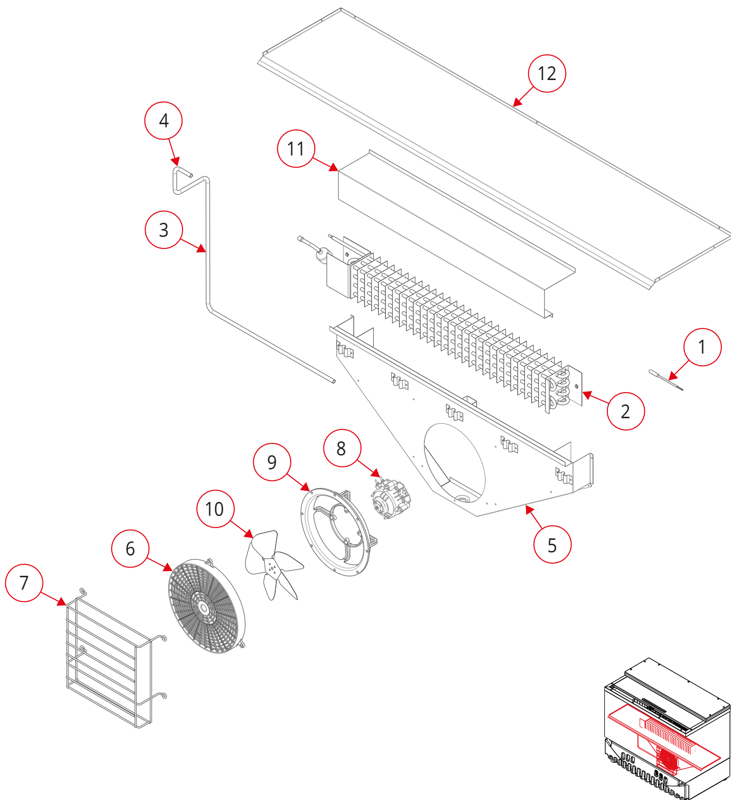
ENSAMBLE EVAPORADOR
