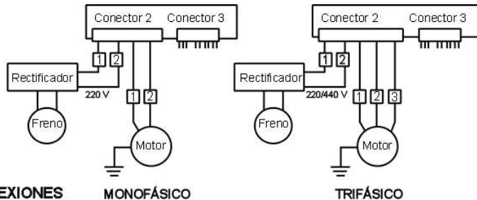
FIG. A2 CONEXIONES
