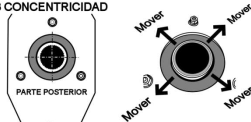
FIG. A3 CONCENTRICIDAD
