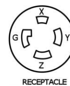
RECEPTACLE
